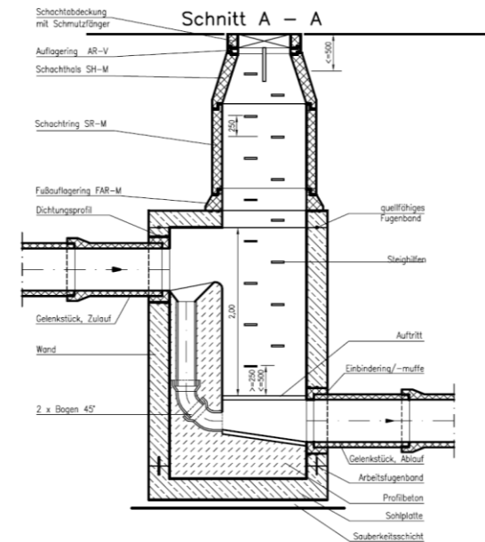
Absturzbauwerk in der Kanalisation
